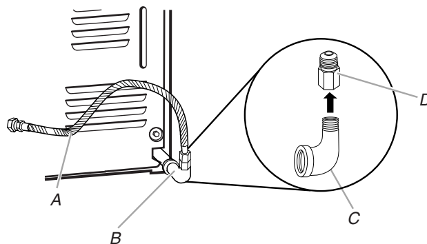
A. Conector flexible de gas de \frac{3}{8} "
